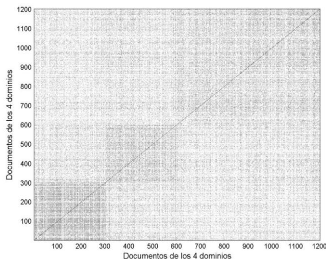
Fig. 5. Gráfica de similitud
