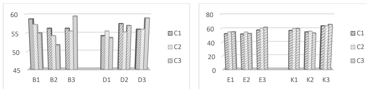
Fig. 4. Resultados usando SVM
